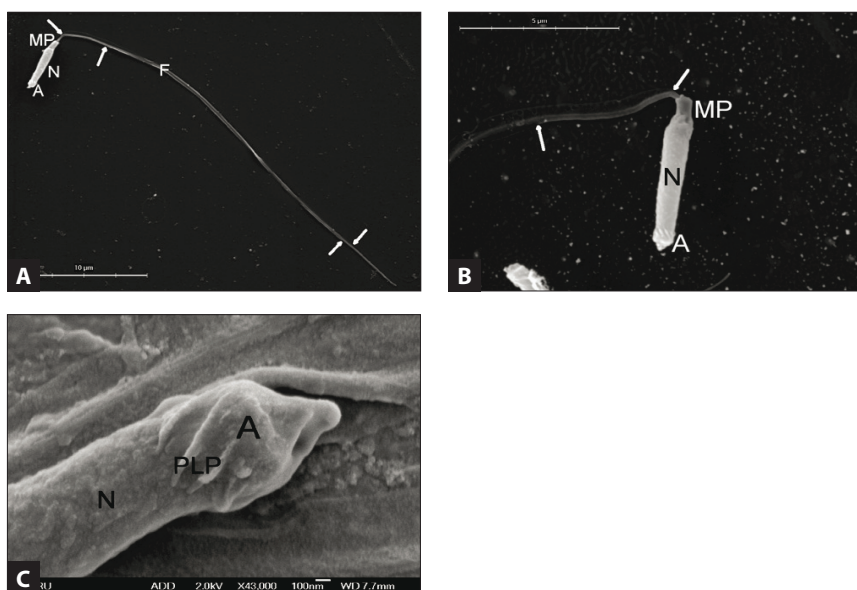
Obr. 1. Ultrastruktura spermie jesetera malého pořízená skenovacím elektronovým mikroskopem (SEM) ukazuje na obrázku a) celou spermii (měřítko 10 μm), šípky vyznačují začátek a konec lemu na bičíku; na obrázku b) větší detail hlavičky spermie, střední části s částí bičíku (měřítko 5 μm) a na obrázku c) s detailem akrozomu na hlavičce spermie (měřítko 100 nm). Akrosom (A), jádro – nukleus (N), střední část (MP), bičík (F), Pšenička a kol. 2009).
