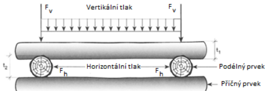
Obr. 9 Statické řešení srubových stupňů Zdroj: Holzkonstruktionen im Wildbach-, Hang-und Runsenverbau. [8]
