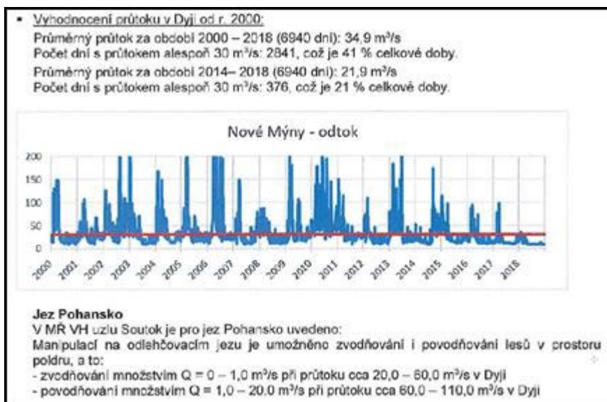
Obr. 8 Průměrné průtoky v Dyji; průtoky v náпустném objektu Pohansko v závislosti na průtocích v Dyji (Povodí Moravy, 2019).
