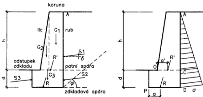
Obr. 2 Tlak zeminy na opěrnou zeď. Zdroj:
