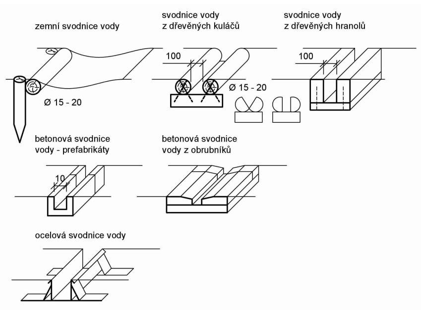
Obr. 3 Typy svodnic vody – převzato: [6]
