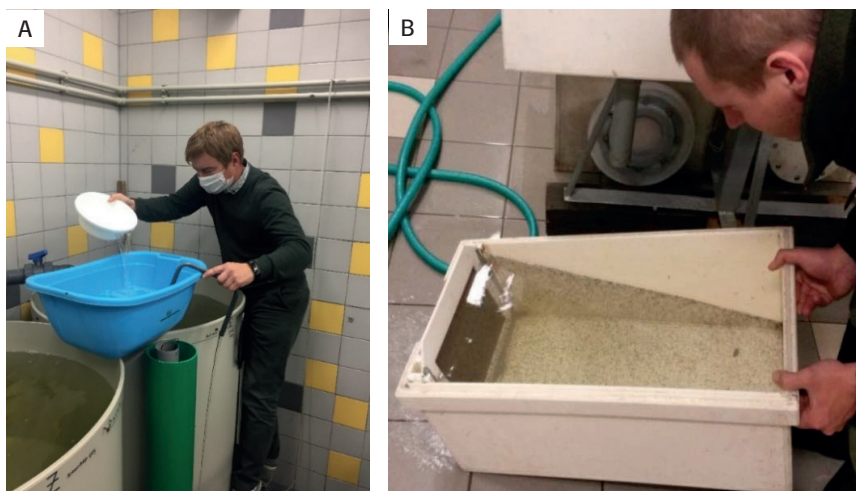
Obr. 20. Odebírání larev z inkubační nádrže (A) a zahušťování larev v líhňarské kolíbkce (B) u candáta obecného ( Sander lucioperca ) (Foto T. Polícar).
