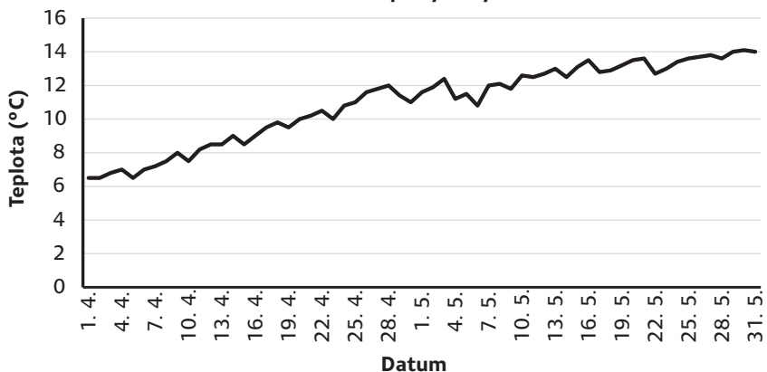
Obr. 13. Procentuální podíl jednotlivých stadií oocytů a procentuální četnost výtěrů v jednotlivých období reprodukční sezóny u 180 použitých generačních samic candáta obecného ( Sander lucioperca ) včetně záznamu průběhu teplot.
