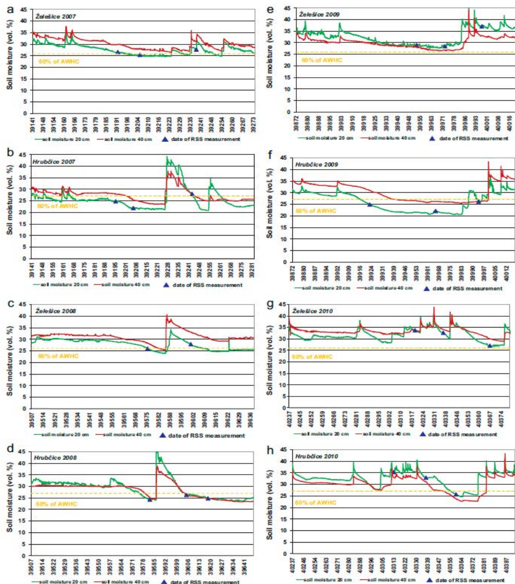
Obr. 12 Vlhkost půdy pod porostem pšenice v hloubkách 20 a 40 cm během vegetačního období (březen až červenec) v letech 2007–2010 (a – Želešice 2007, b – Hrubčice 2007, c – Želešice 2008, d – Hrubčice 2008, e – Želešice 2009, f – Hrubčice 2009, g – Želešice 2010, h – Hrubčice 2010). Časové měřítko na osách X je uvedeno v číselném formátu pro možnost jeho použití ve výpočtech, když pořadové číslo dne se v aplikaci MS Excel načítá od 1. 1. 1900.
